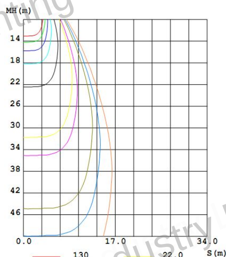
均等な平面照度図
