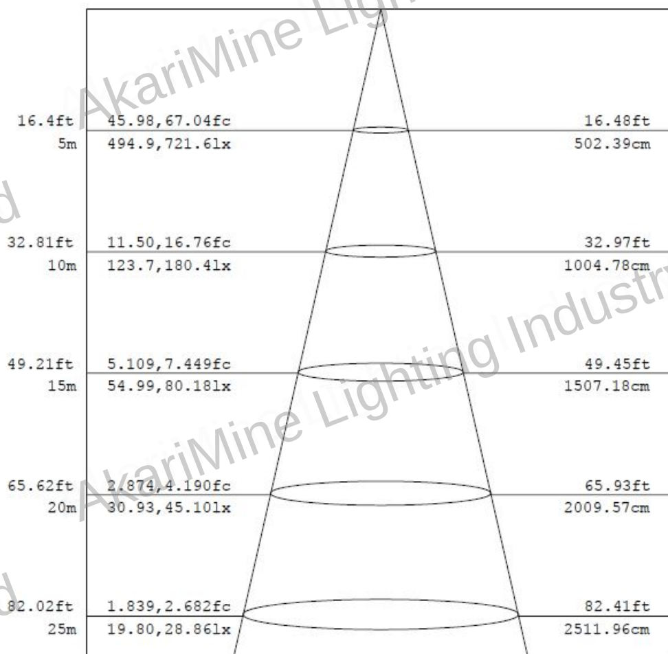
垂直照度図
